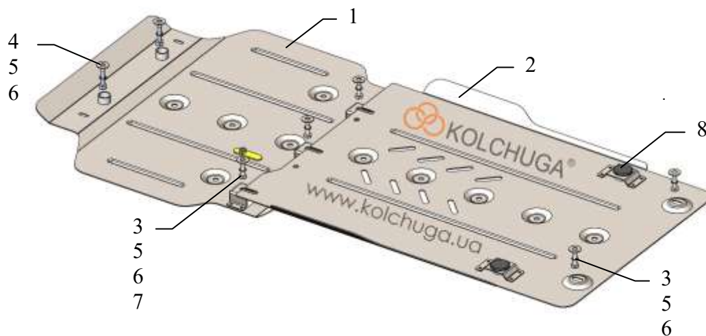
Схема захисту.
