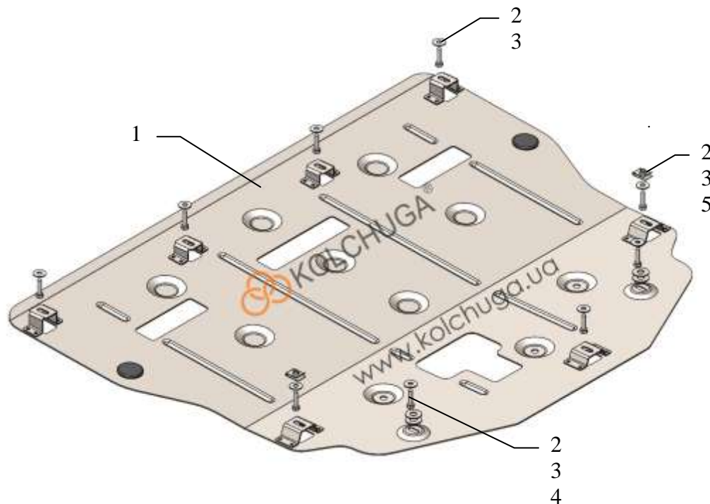
Схема захисту.
