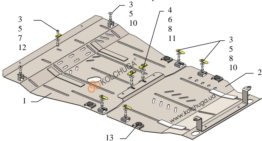
Схема сборки.
