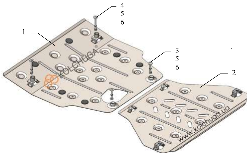
Схема сборки.
