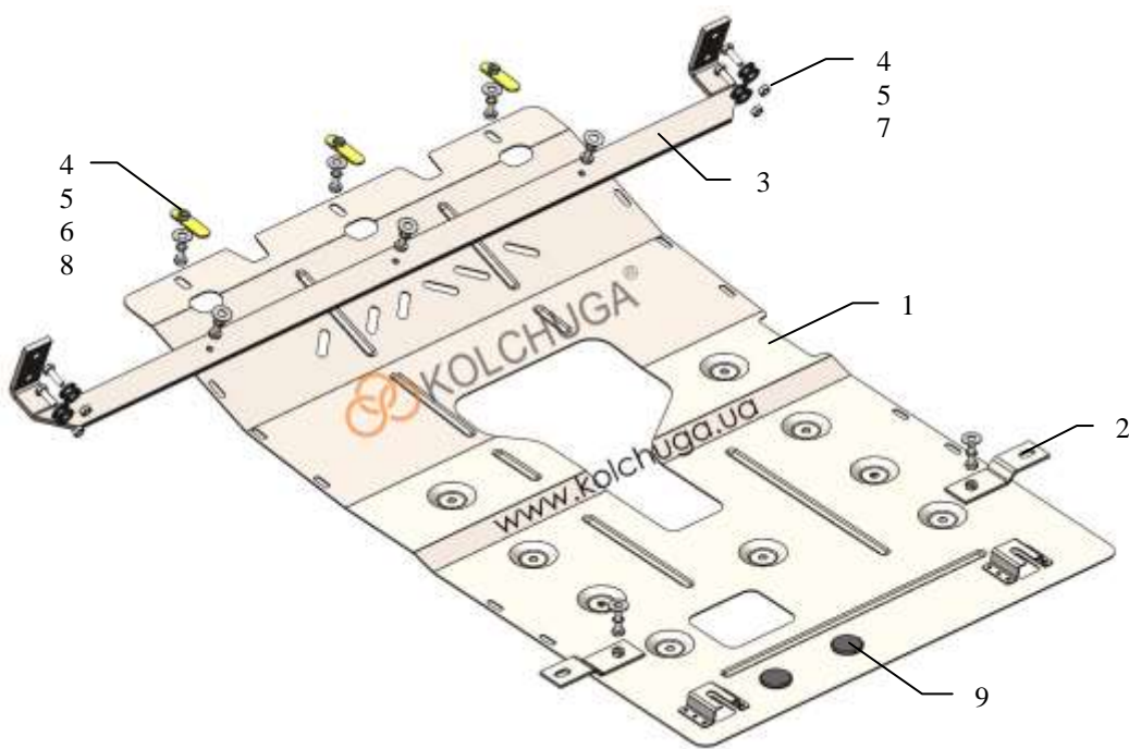
Схема захисту.
