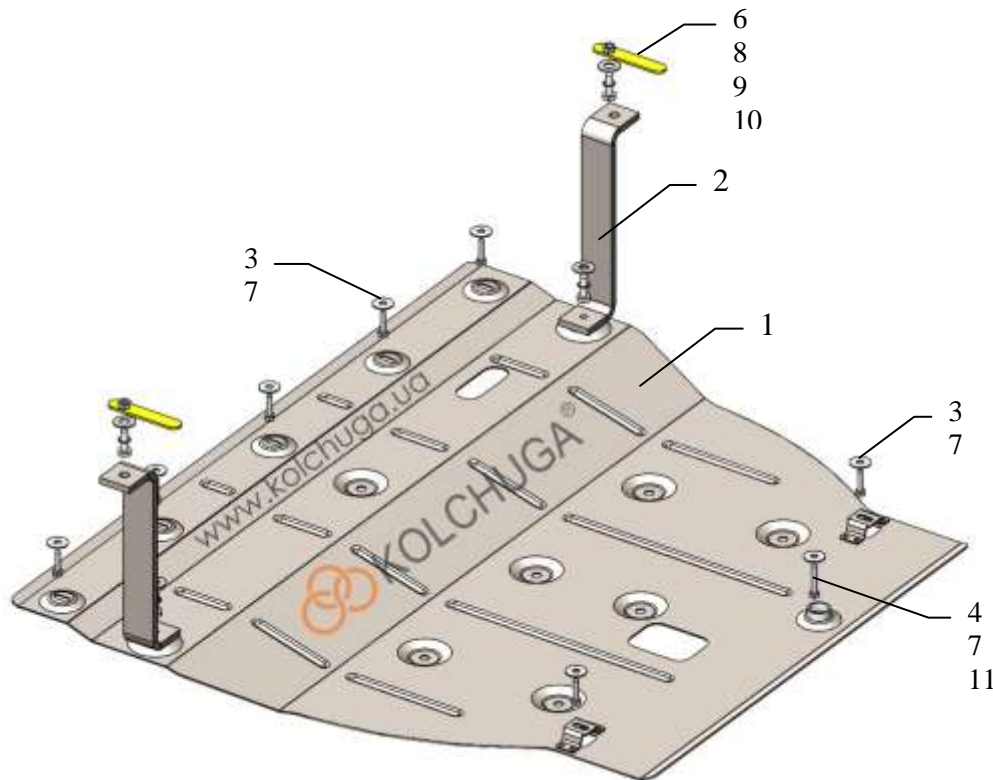
Схема збірки захиста.
