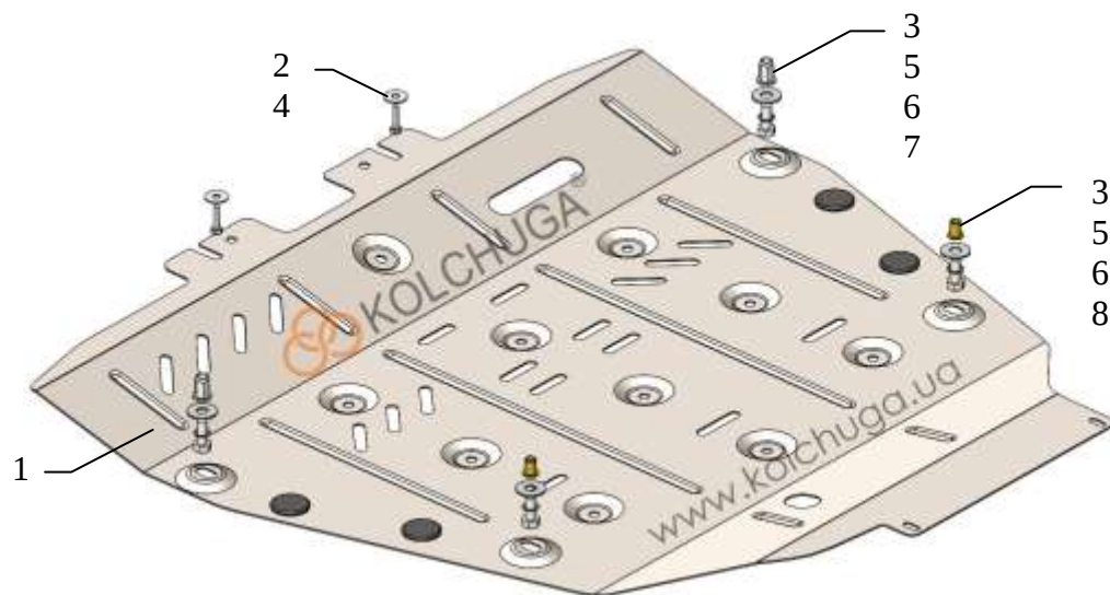
Схема збірки.
