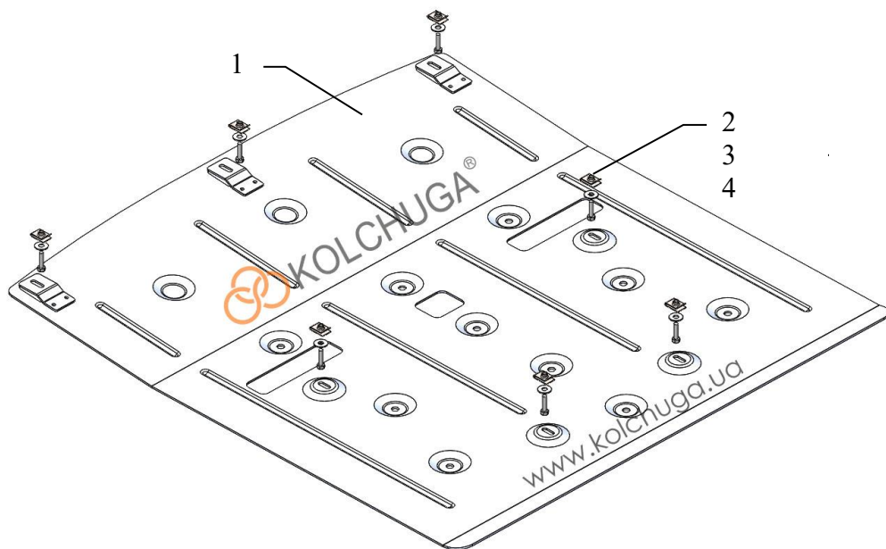
Схема захисту.
