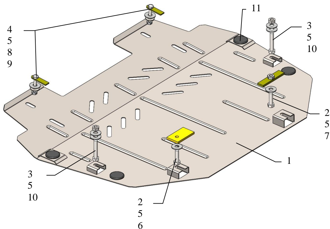
Схема сборки.
