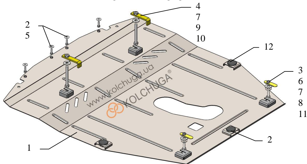
Схема сборки защиты картера и КПП.
