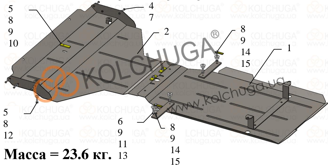
Схема сборки защиты радиатора, двигателя, КПП
