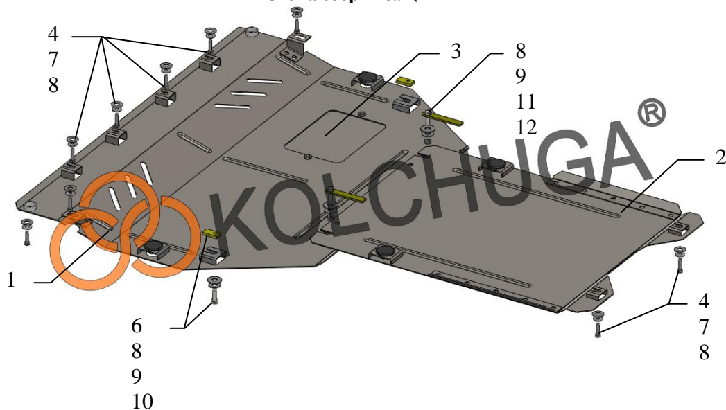
Схема сборки защиты
