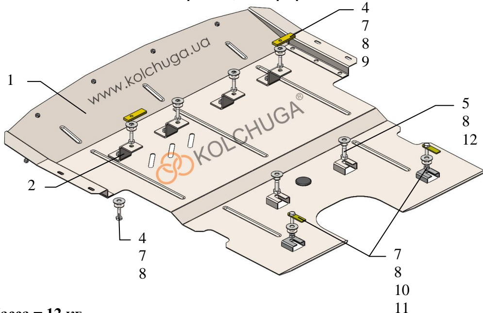
Схема сборки защиты картера и КПШ.
