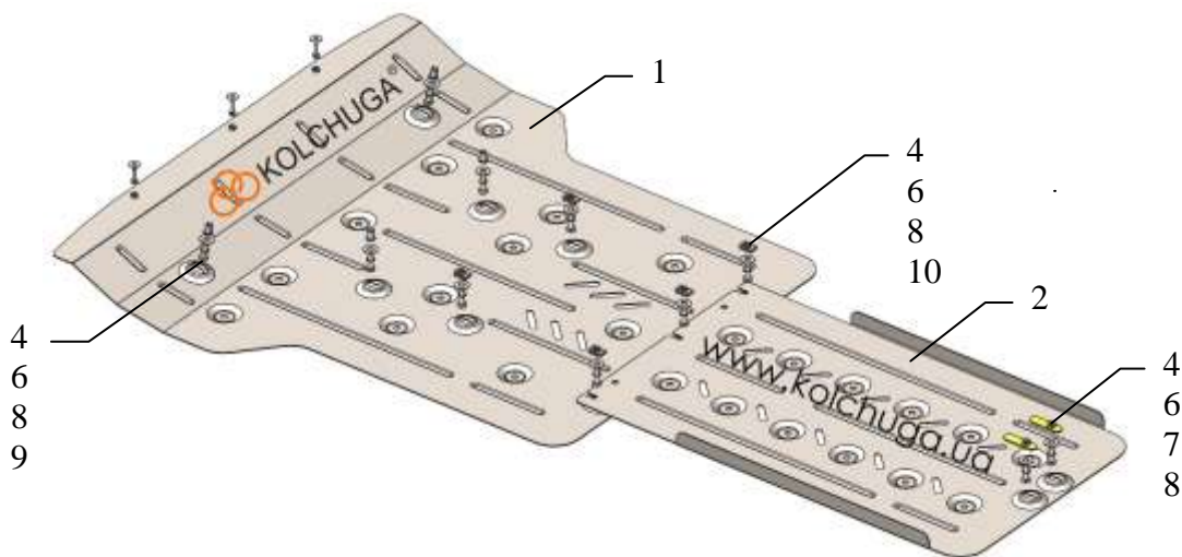
Схема сборки.
