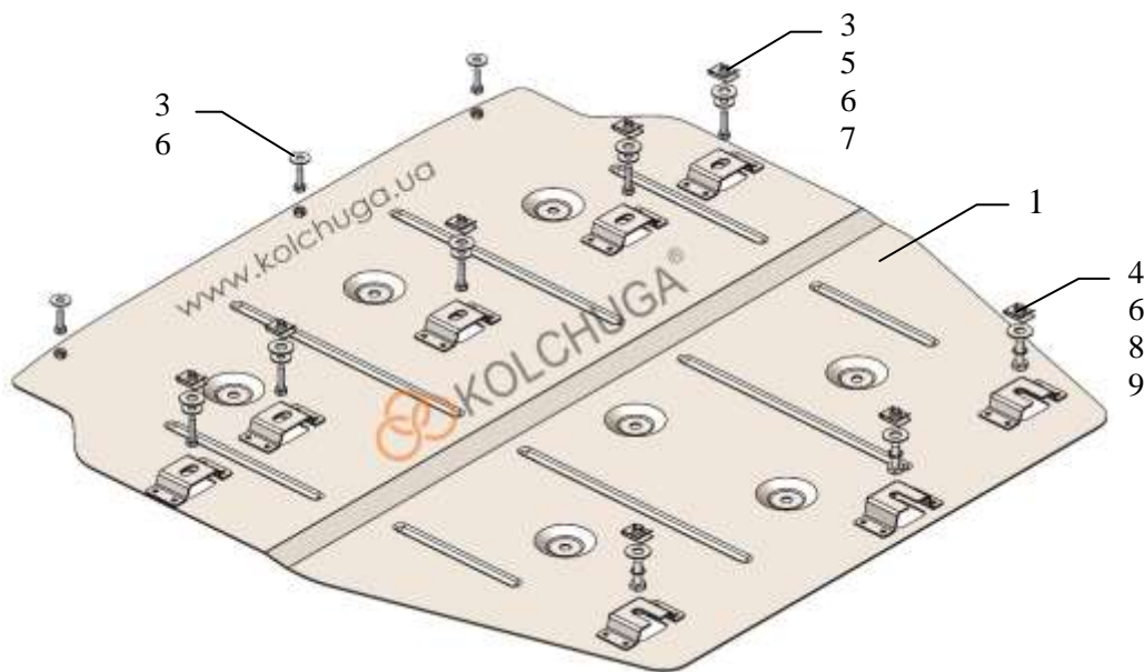
Схема захисту.
