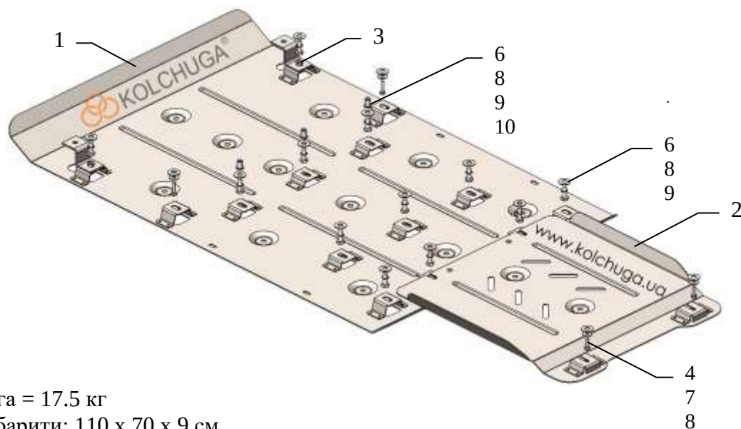
Схема захисту.
