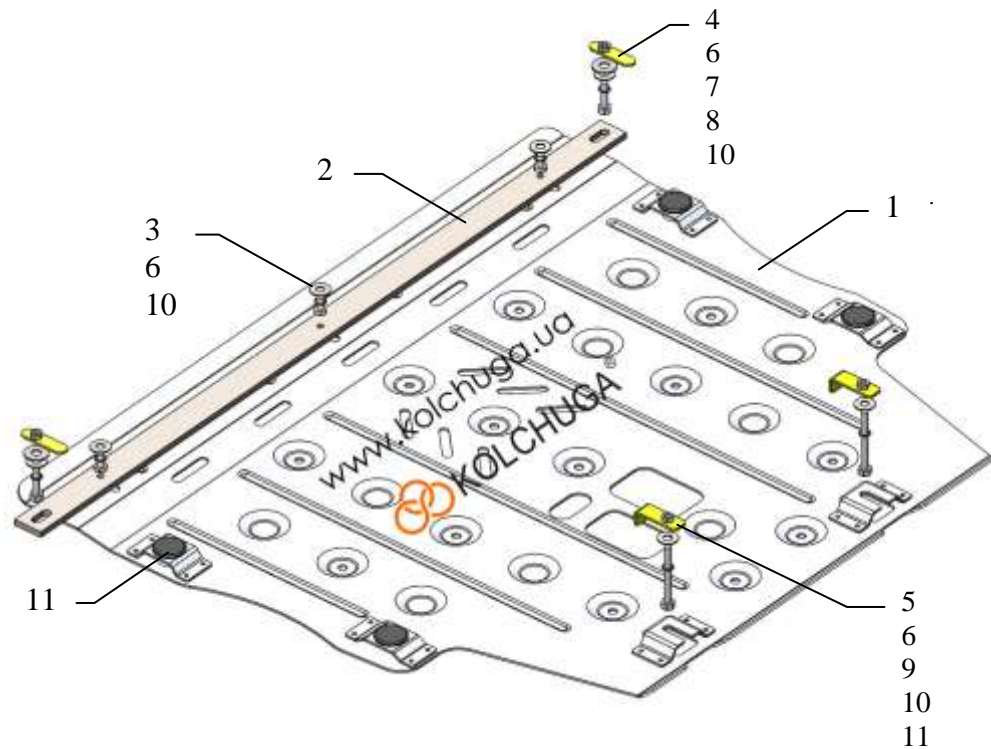
Схема сборки.
